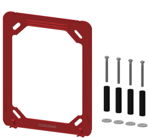
Rama montażowa
