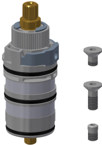
Termoelement 2030003300 EAQLT0004
